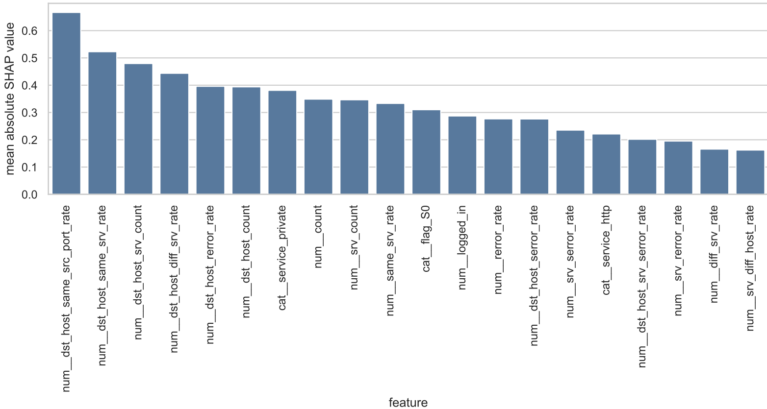
normal: Mean Absolute SHAP Values
